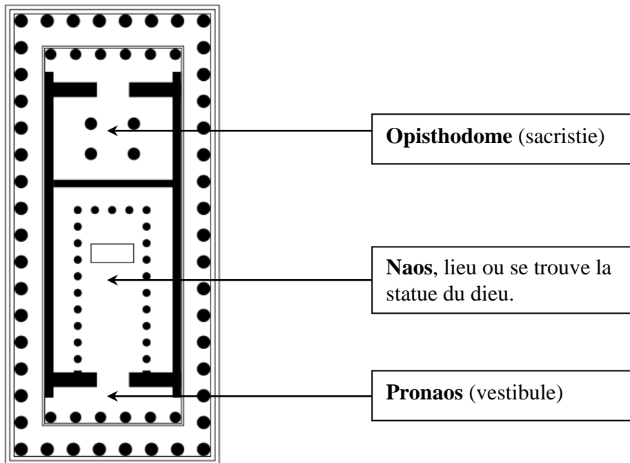
Plan au sol du Parthénon à Athènes, VI e -V e siècles
